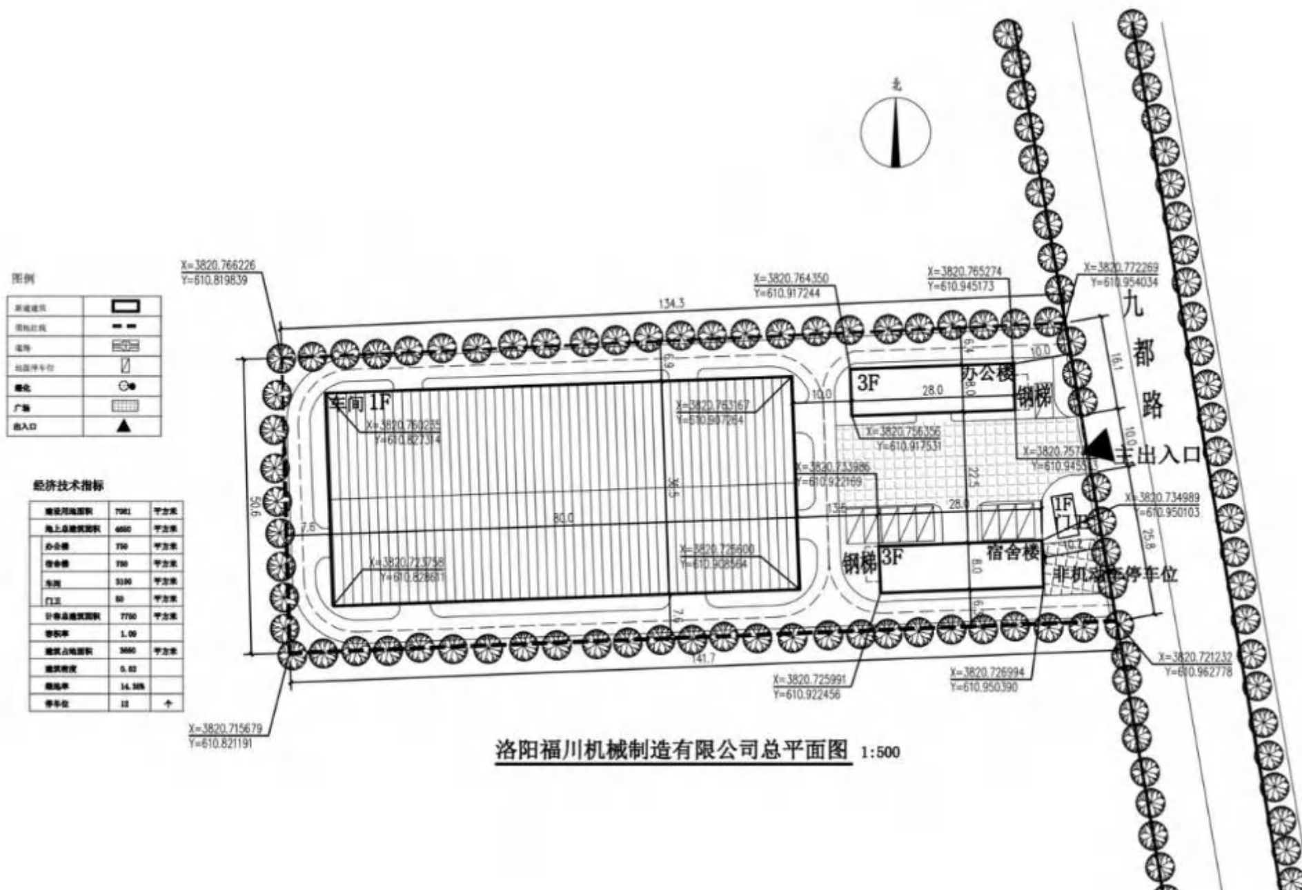
附图 4 厂区总平面布置图
