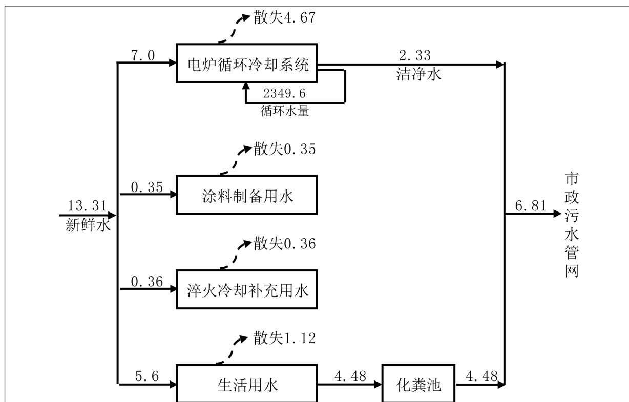
图 1 项目用排水平衡图 单位: t/d
